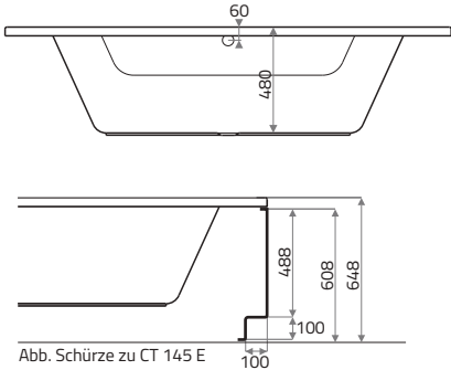
Abb. Schürze zu CT 145 E
